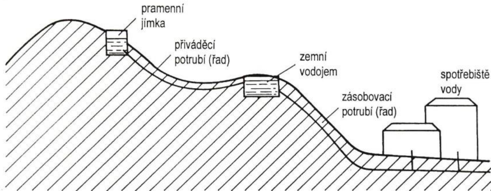
Gravitační (samospádový) vodovod
