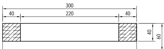
Řez A
