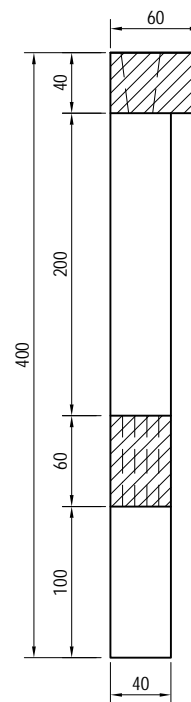
Řez B
