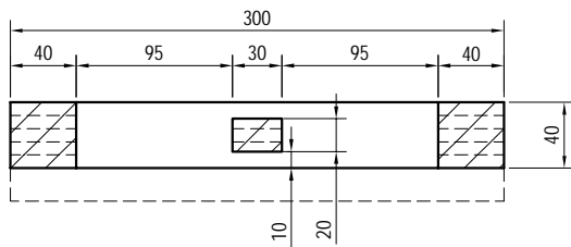
Řez A
