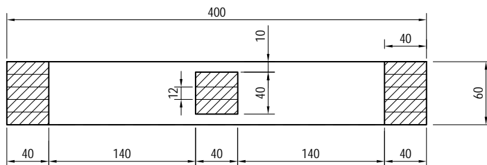
Řez A
