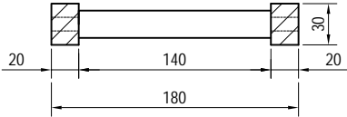
Řez C
