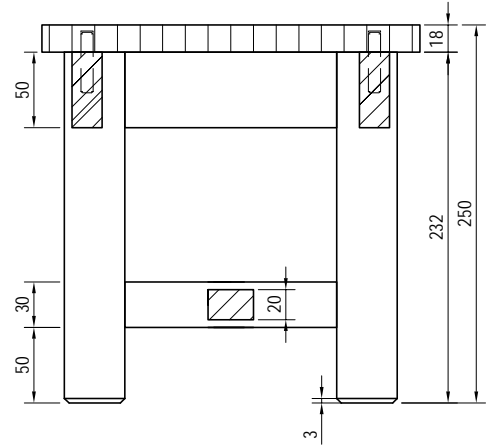
Řez B-B
