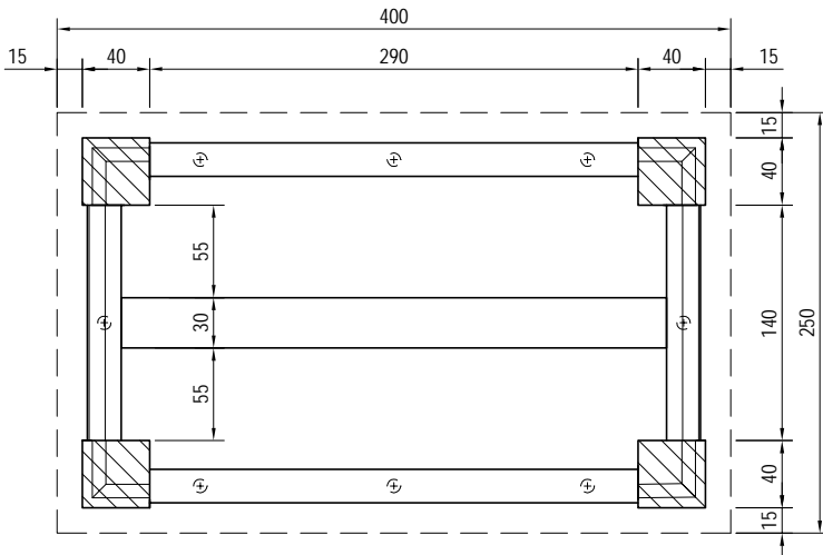
Řez A-A
