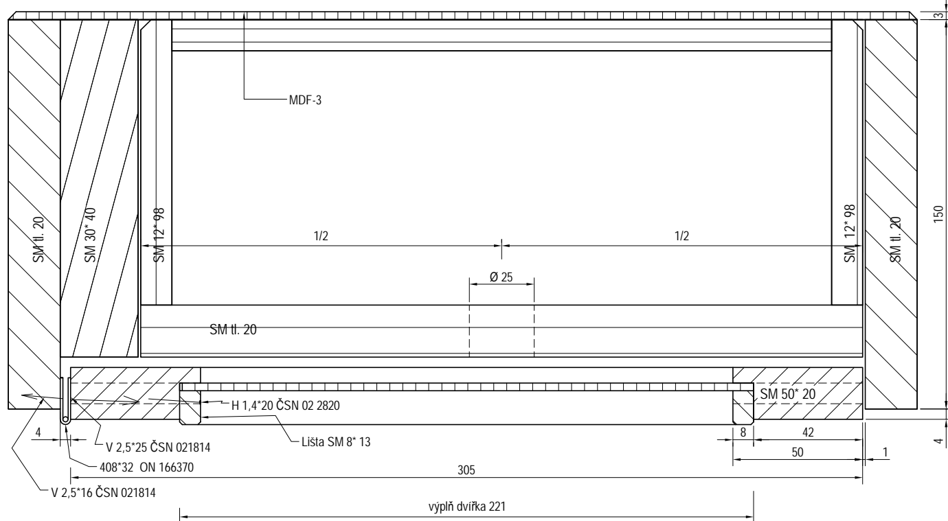
Řez A-A m: 1:2
