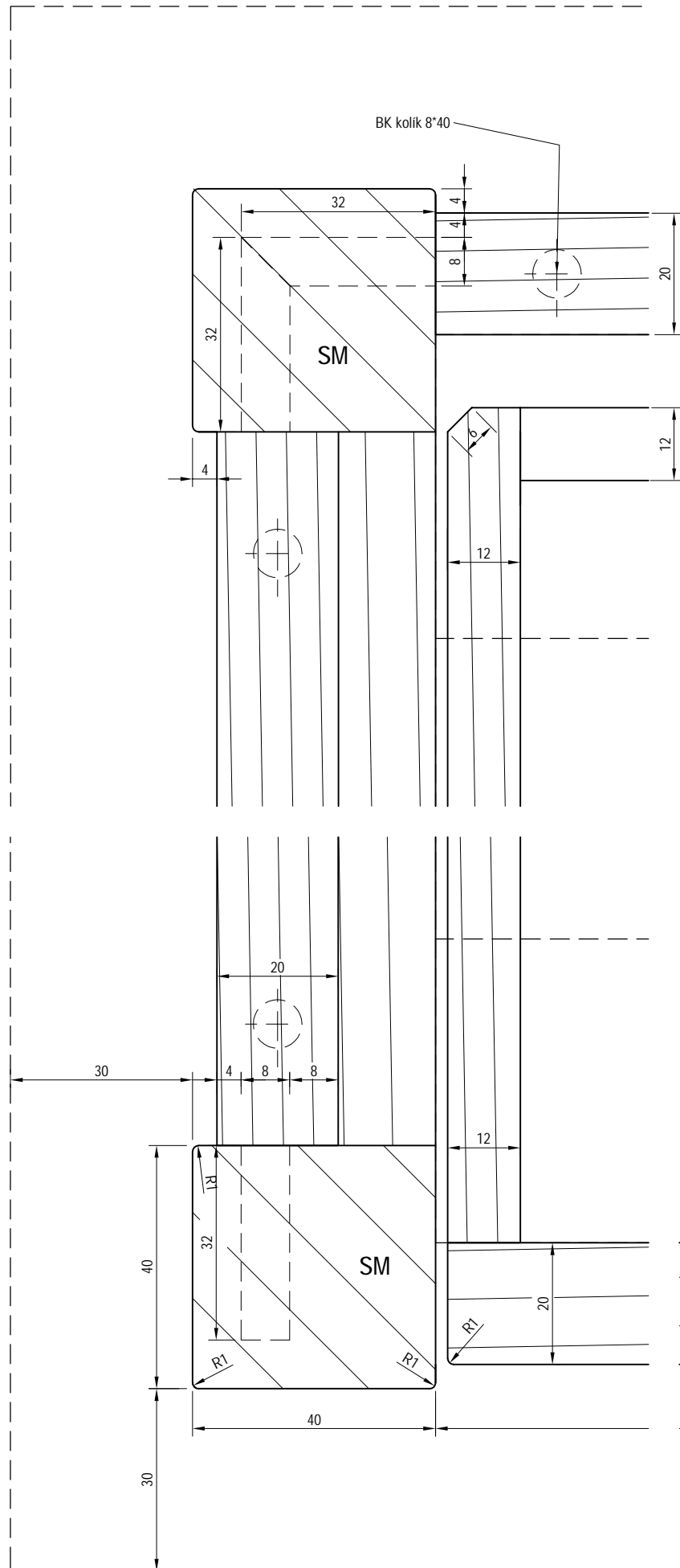
Detail řezu A-A, m: 1: 1
