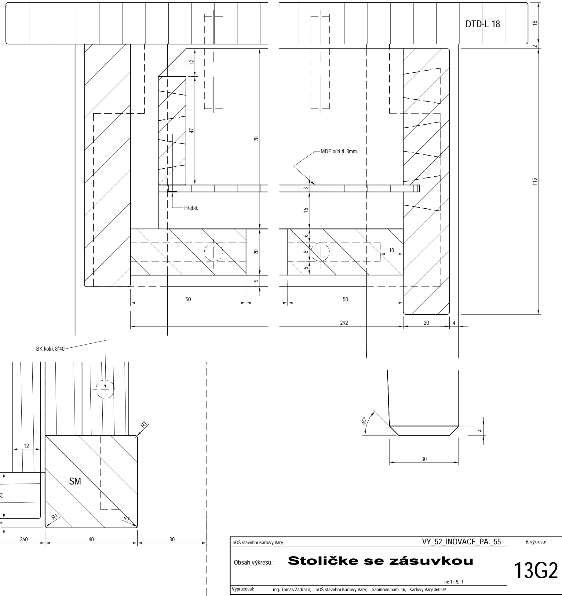
Detail řezu B-B, m: 1: 1
